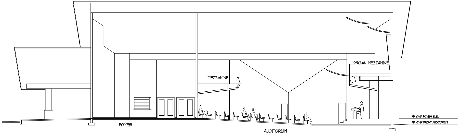
LONGITUDINAL SECTION THRU AUDITORIUM
